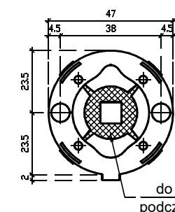
Widok z dołu rozeta montażowa II element b
