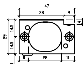
Widok z przodu rozeta montażowa II
