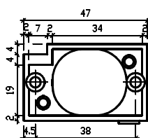
Widok z tyłu rozeta montażowa II
