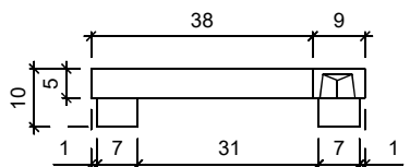
Widok z boku rozeta montażowa II
