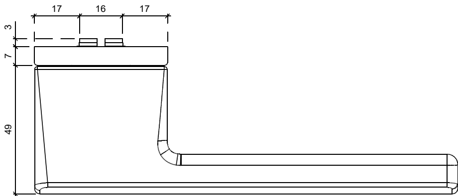
Widok z góry klamka I
