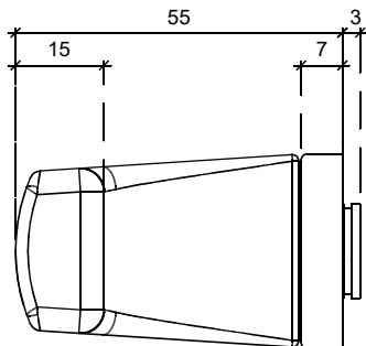
Widok z prawej strony klamka I
