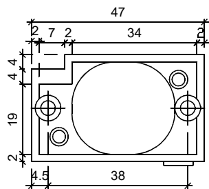
Widok z tyłu rozeta montażowa II
