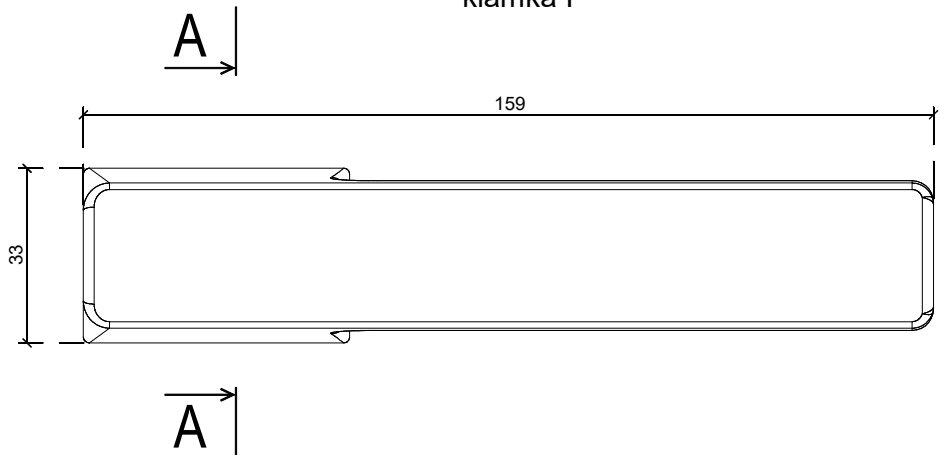
Widok z przodu klamka I
