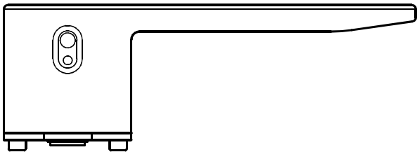
Widok z góry klamka I (wariant z zamkiem)
