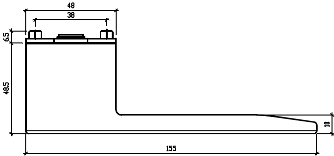
Widok z góry klamka I
