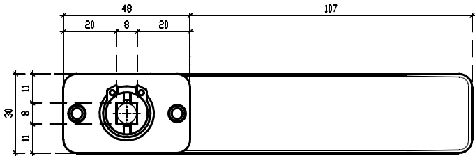
Widok z tyłu klamka I
