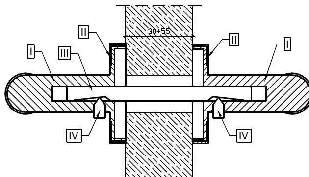
Schemat montażu elementów Przekrój A-A
