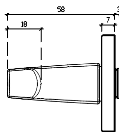
Widok z prawej strony klamka I
