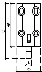
Widok z przodu stoper I
