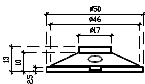
Widok z przodu stoper III
