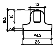
Widok z góry stoper I
