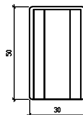
Widok z tyłu stoper II
