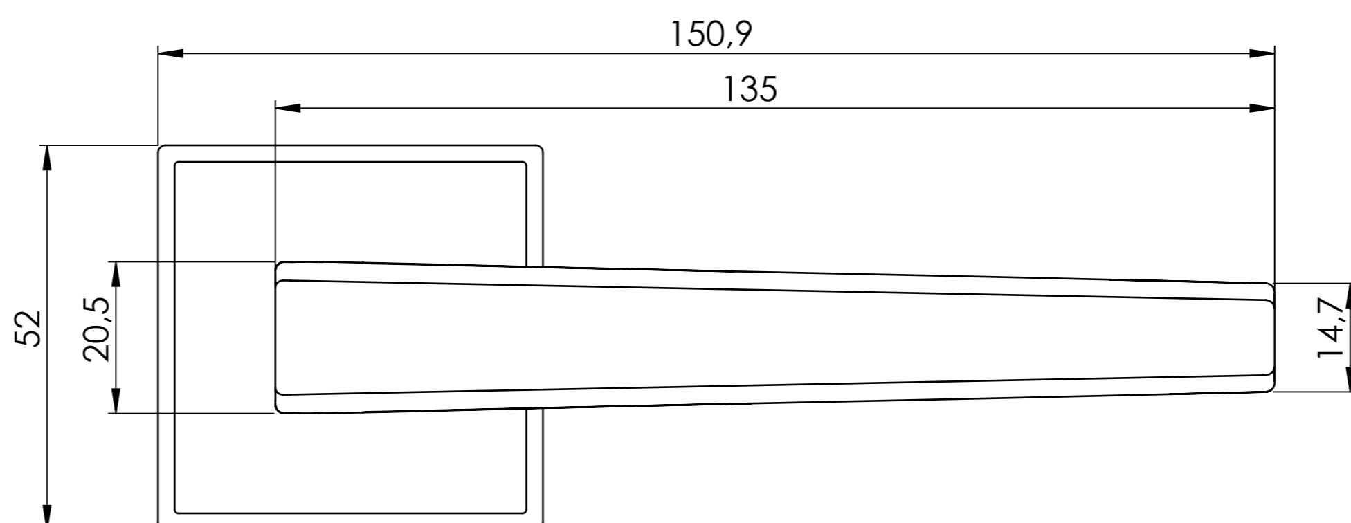
Widok z przodu Klamka I
