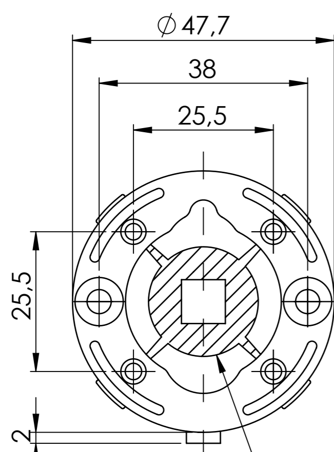
Widok z przodu Rozeta montażowa II
